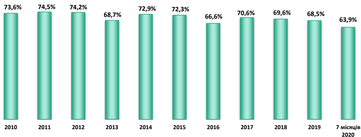
Рис.3. Коефіцієнт використання встановленої потужності енергоблоків АЕС
