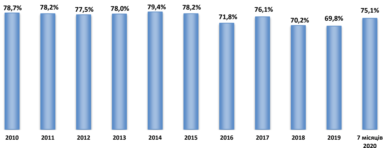
Рис.4. Коефіцієнт готовності несення номінального електричного навантаження АЕС
